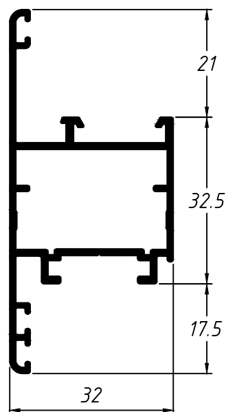
Folha perimetral abertura externa MT337 0,910Kg/m
