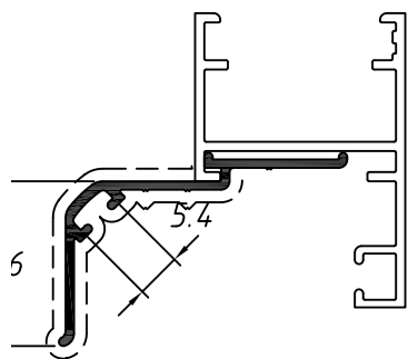
Pingadeiro IN055 0,173 Kg/m
