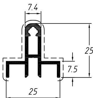
Marco 1 trilho multifunção IN104 0,364 Kg/m
