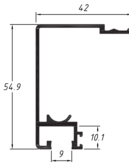
Guía superior leve para 8mm LGGS 0,547 Kg/m
