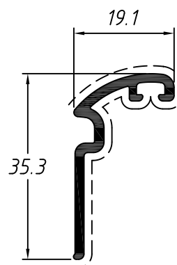
Tampa junta IN203 0,278 Kg/m
