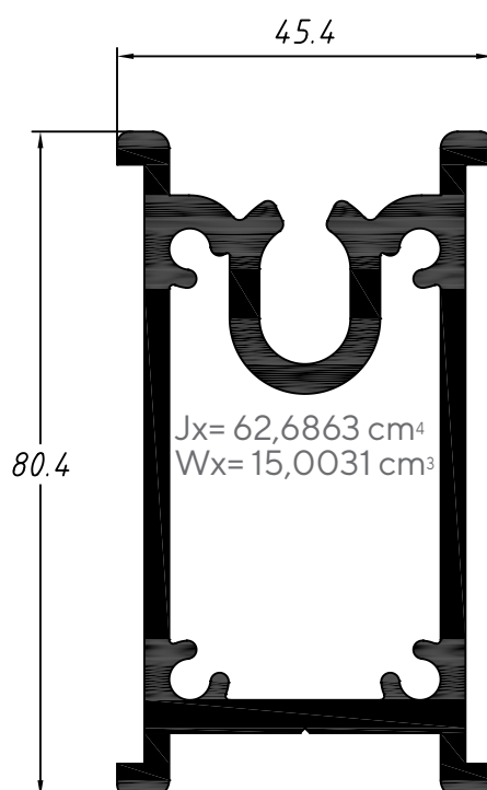
Reforço interno fc017 e fc200 FC018 2,645 Kg/m
